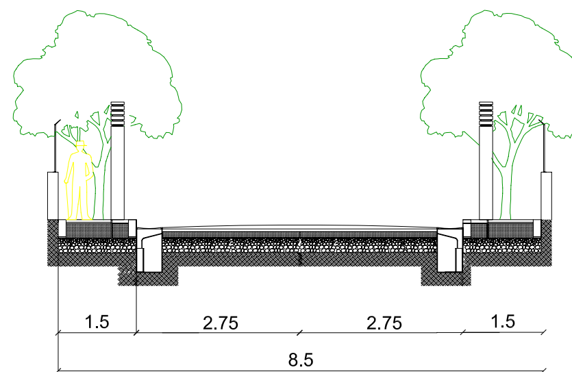
SEZIONE STRADALE 2
