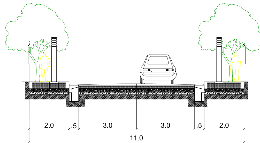
SEZIONE STRADALE 1
