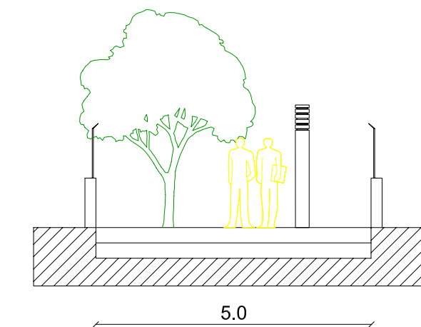
PERCORSO PEDONALE 1
